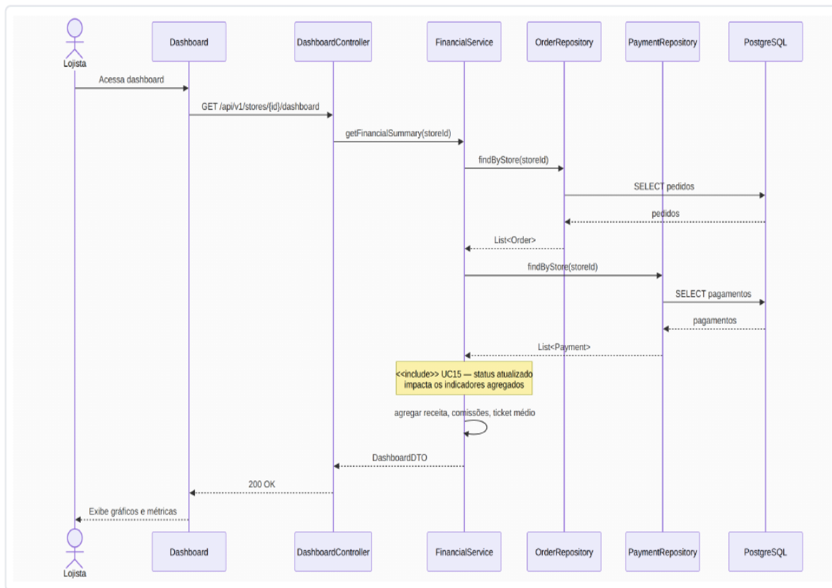
Figura 11 — Diagrama de sequência do UC11 (Visualizar dashboard financeiro).
