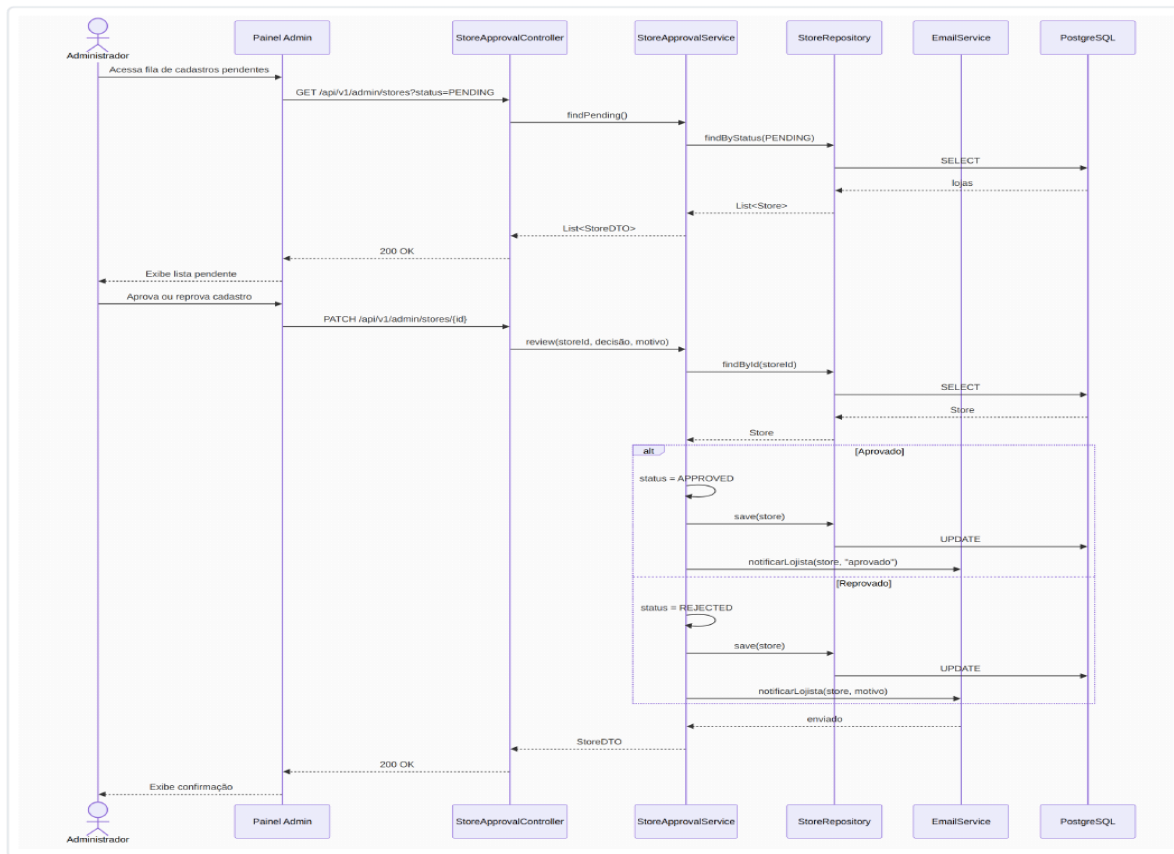
Figura 24 — Diagrama de sequência do UC24 (Aprovar ou reprovar cadastro do lojista).
