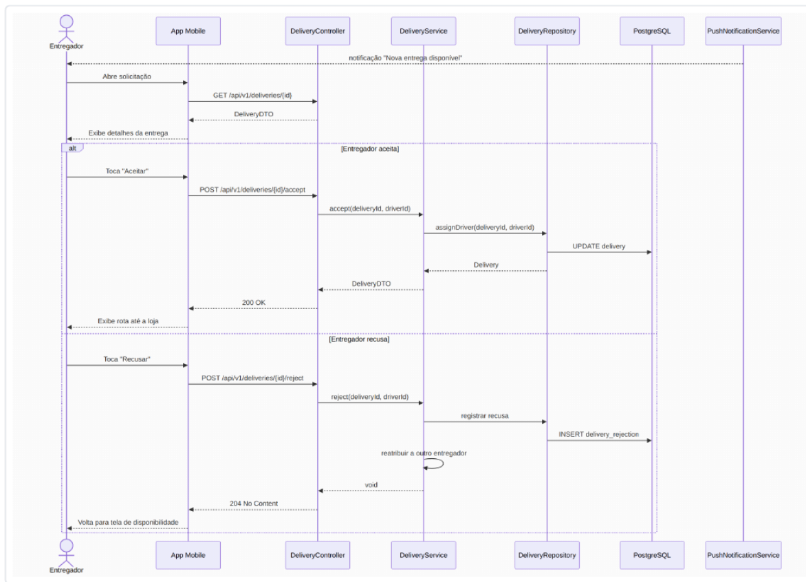
Figura 19 — Diagrama de sequência do UC19 (Aceitar ou recusar entrega).
