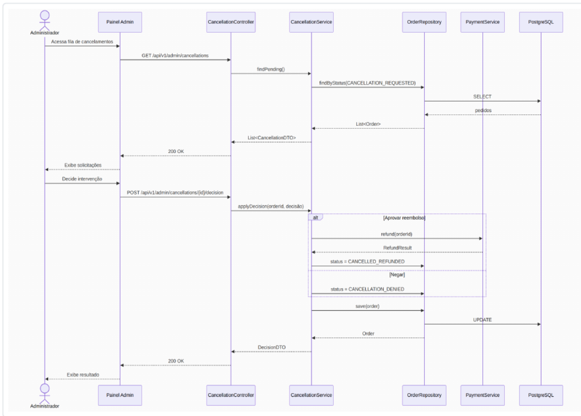
Figura 26 — Diagrama de sequência do UC26 (Intervir em cancelamentos).
