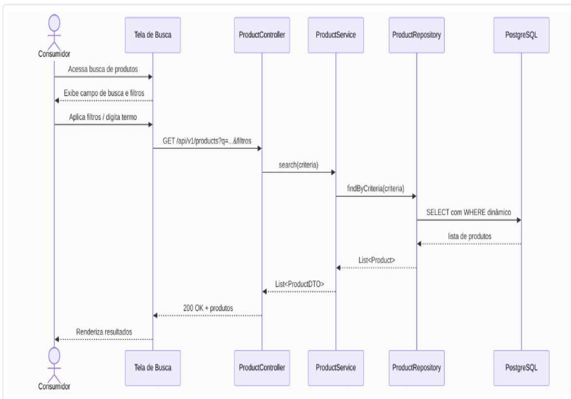
Figura 4 — Diagrama de sequência do UC04 (Buscar e filtrar produtos).
