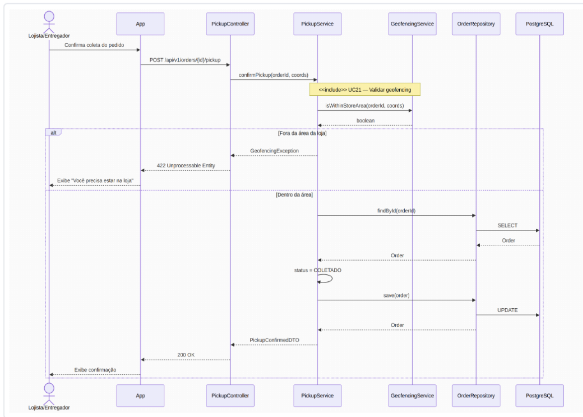
Figura 14 — Diagrama de sequência do UC14 (Confirmar coleta na loja).
