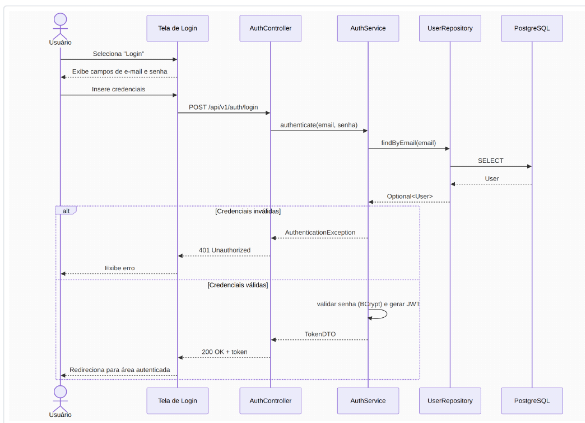
Figura 2 — Diagrama de sequência do UC02 (Fazer login).
