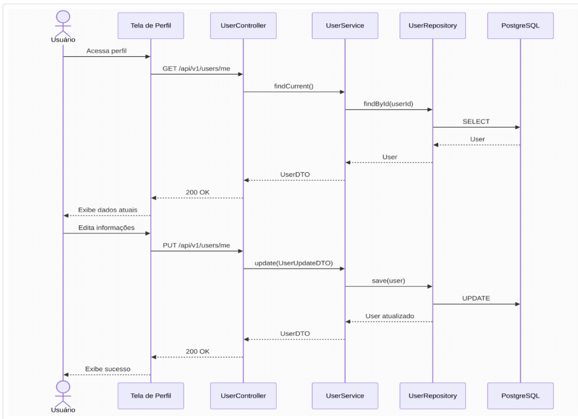
Figura 10 — Diagrama de sequência do UC10 (Gerenciar perfil).
