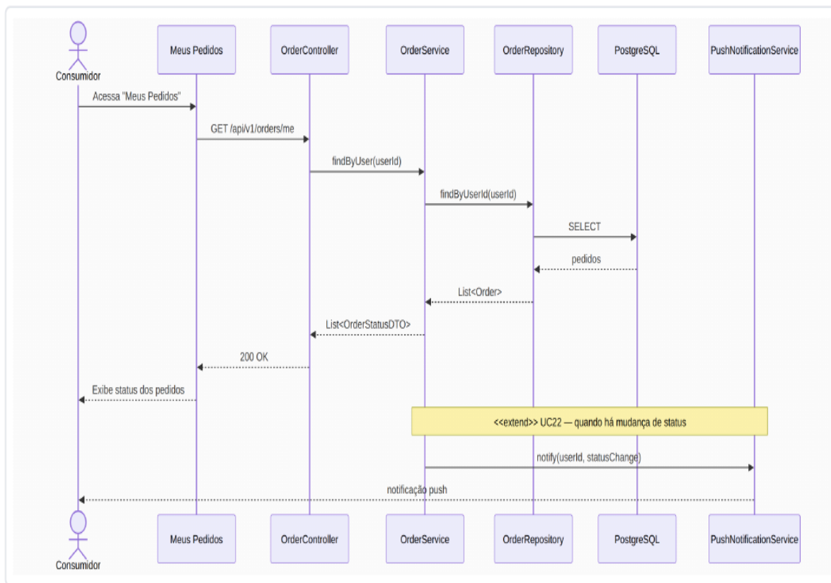
Figura 8 — Diagrama de sequência do UC08 (Acompanhar pedido).
