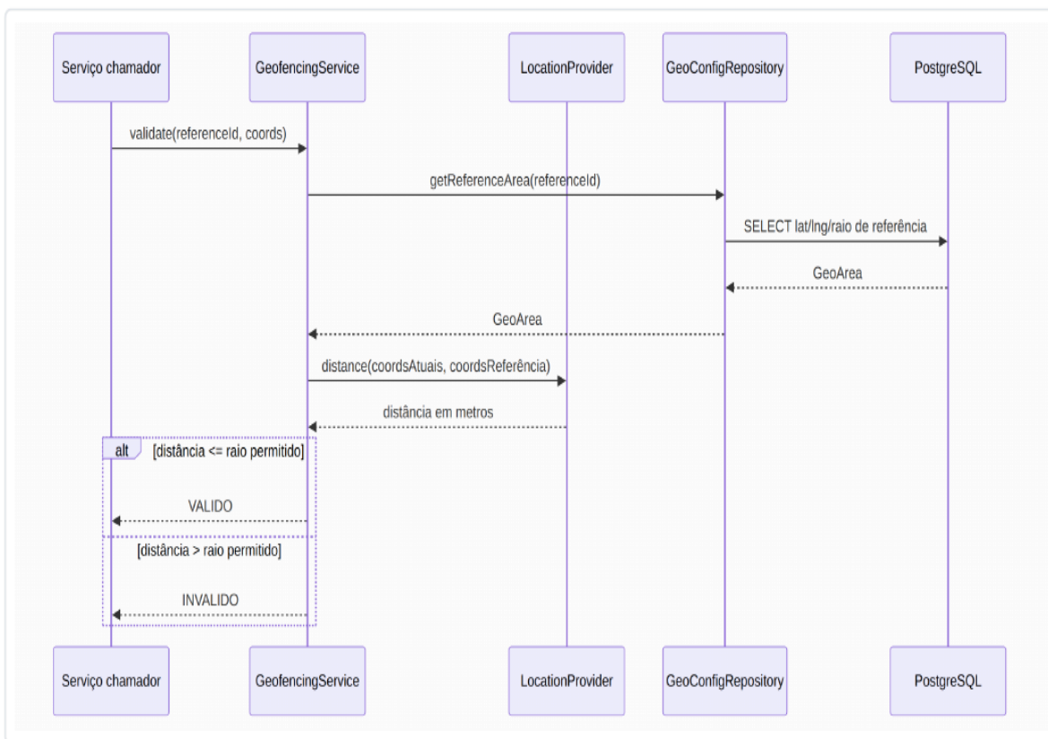
Figura 21 — Diagrama de sequência do UC21 (Validar geofencing).
