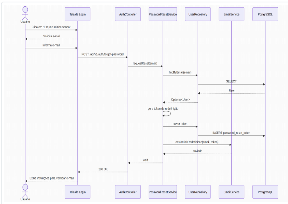
Figura 3 — Diagrama de sequência do UC03 (Recuperar senha).
