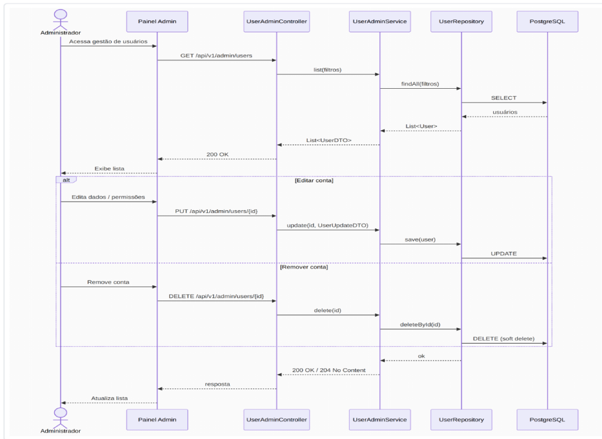
Figura 25 — Diagrama de sequência do UC25 (Gerenciar contas de usuários).
