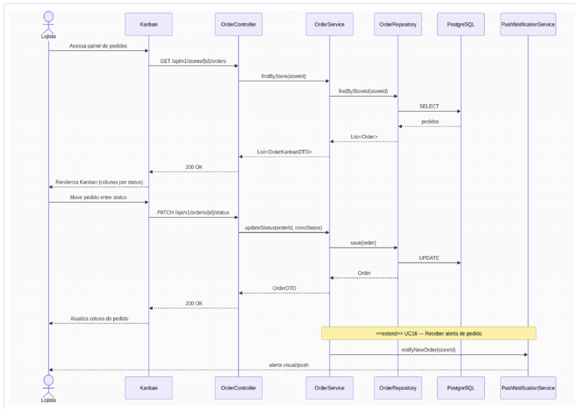
Figura 13 — Diagrama de sequência do UC13 (Gerenciar pedidos (Kanban)).
