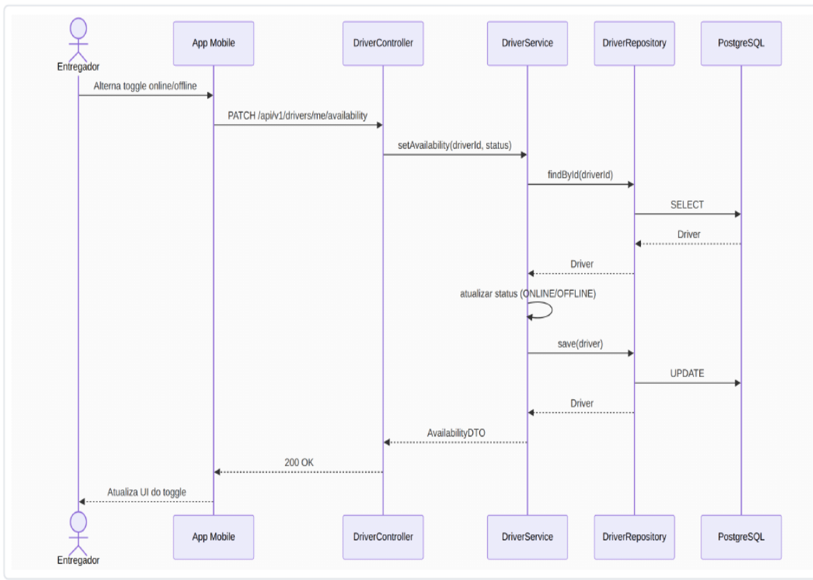
Figura 18 — Diagrama de sequência do UC18 (Alternar disponibilidade online/offline).
