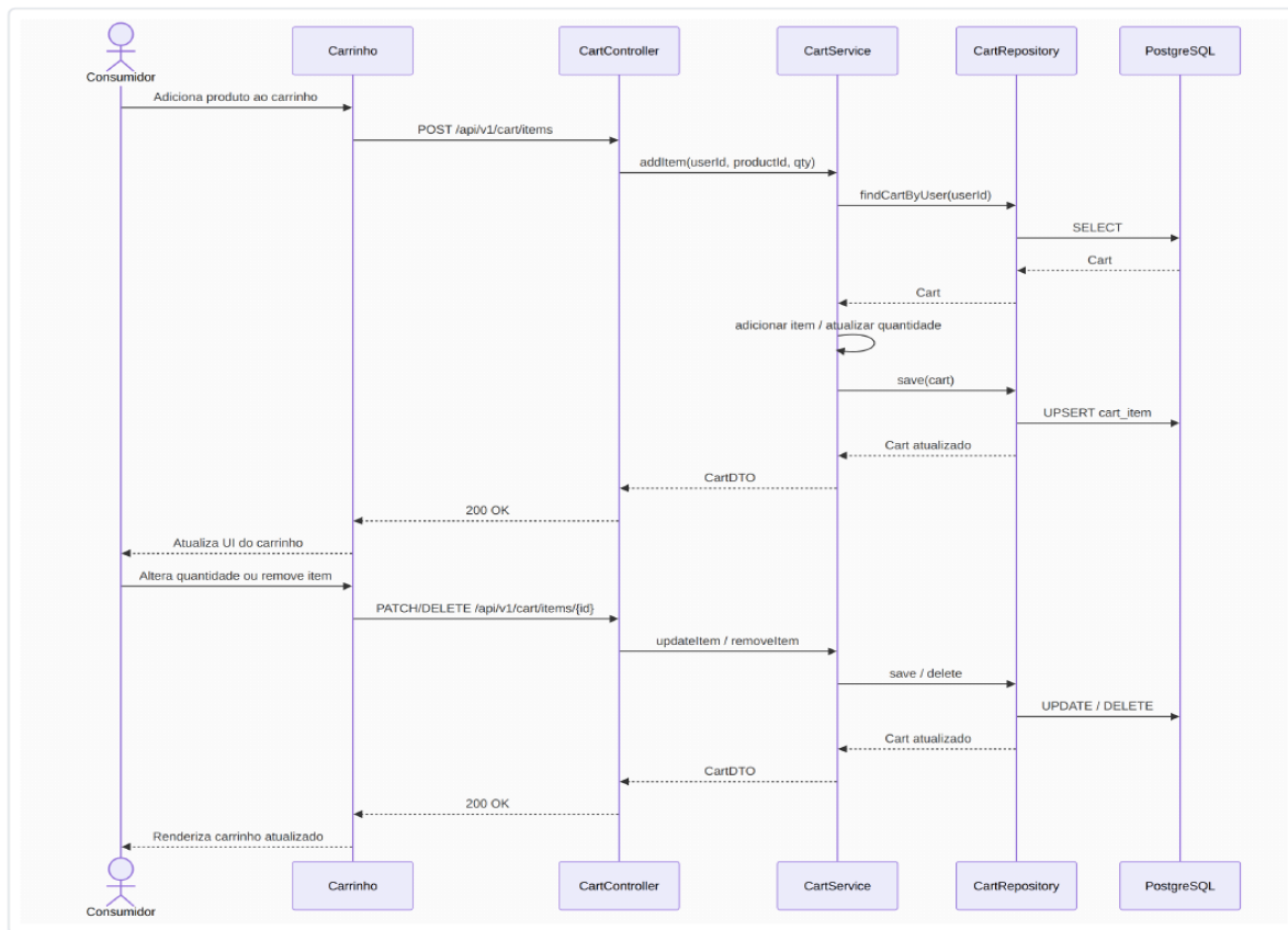
Figura 6 — Diagrama de sequência do UC06 (Gerenciar carrinho).
