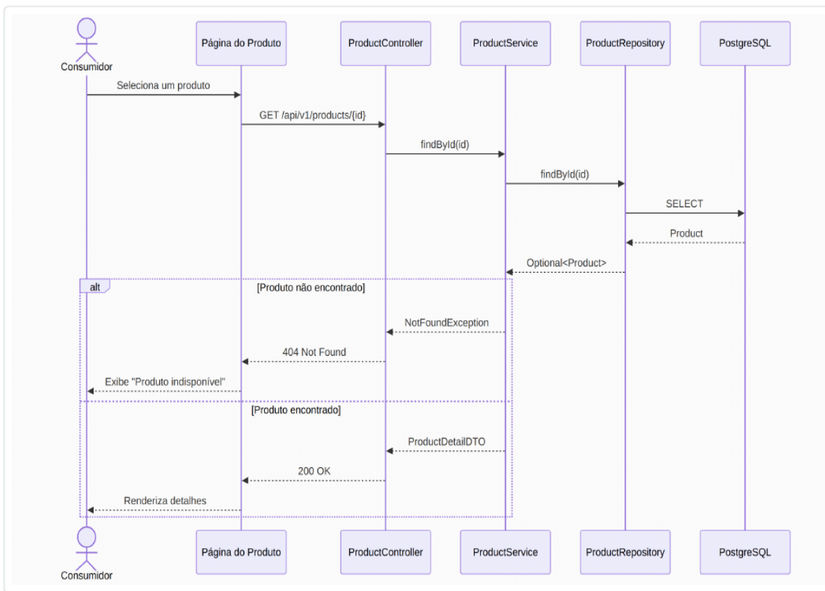
Figura 5 — Diagrama de sequência do UC05 (Visualizar detalhe do produto).
