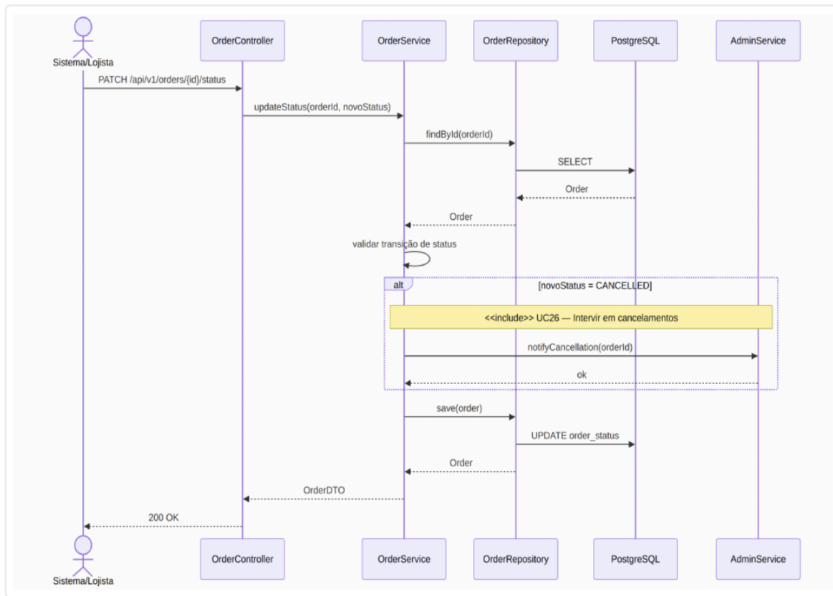
Figura 15 — Diagrama de sequência do UC15 (Atualizar status do pedido).
