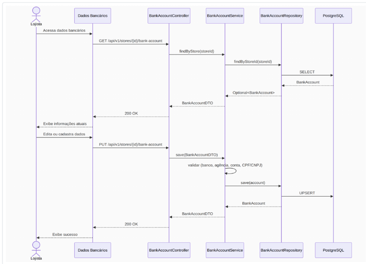
Figura 12 — Diagrama de sequência do UC12 (Gerenciar dados bancários).
