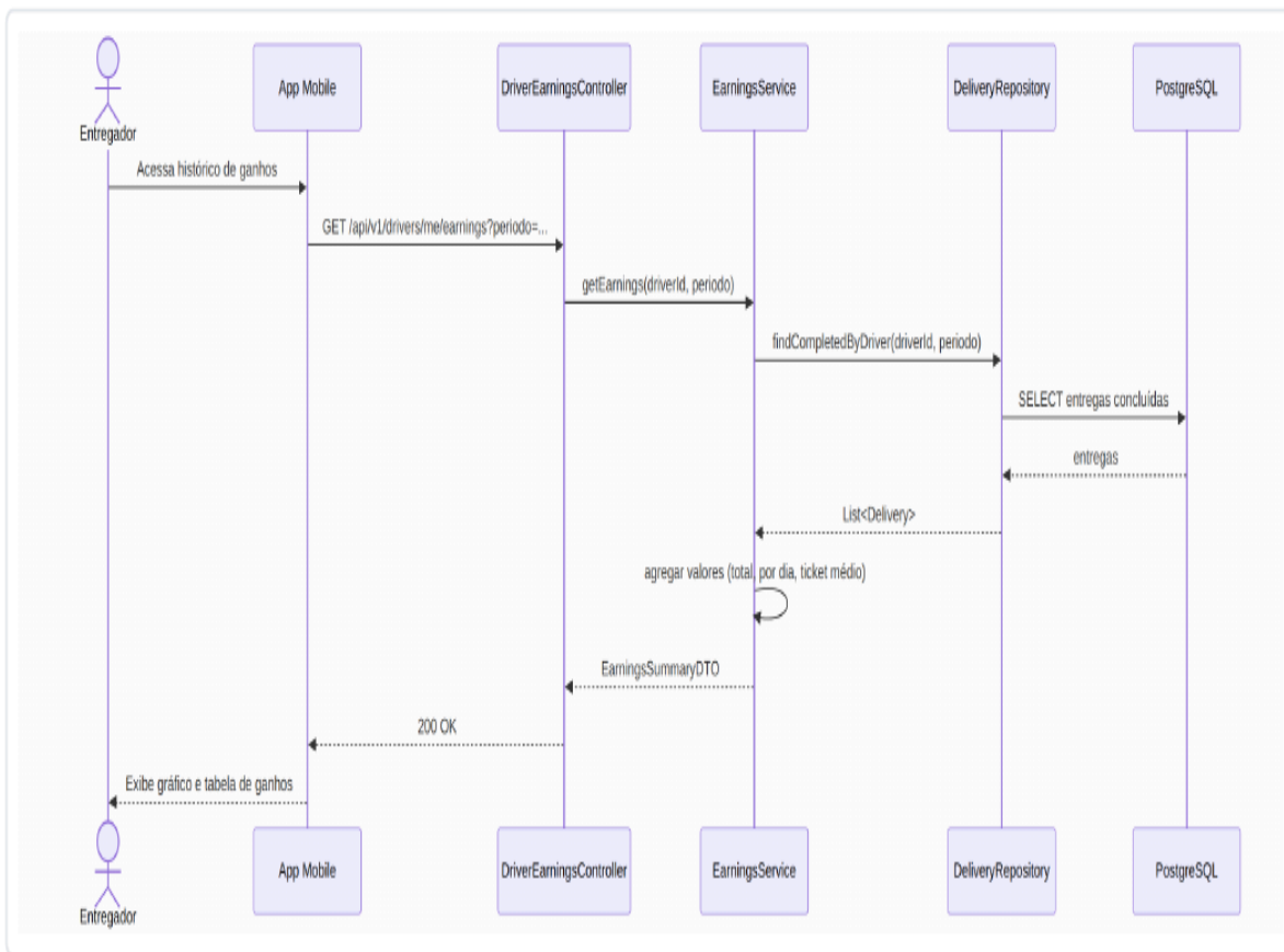
Figura 27 — Diagrama de sequência do UC27 (Consultar histórico de ganhos).
