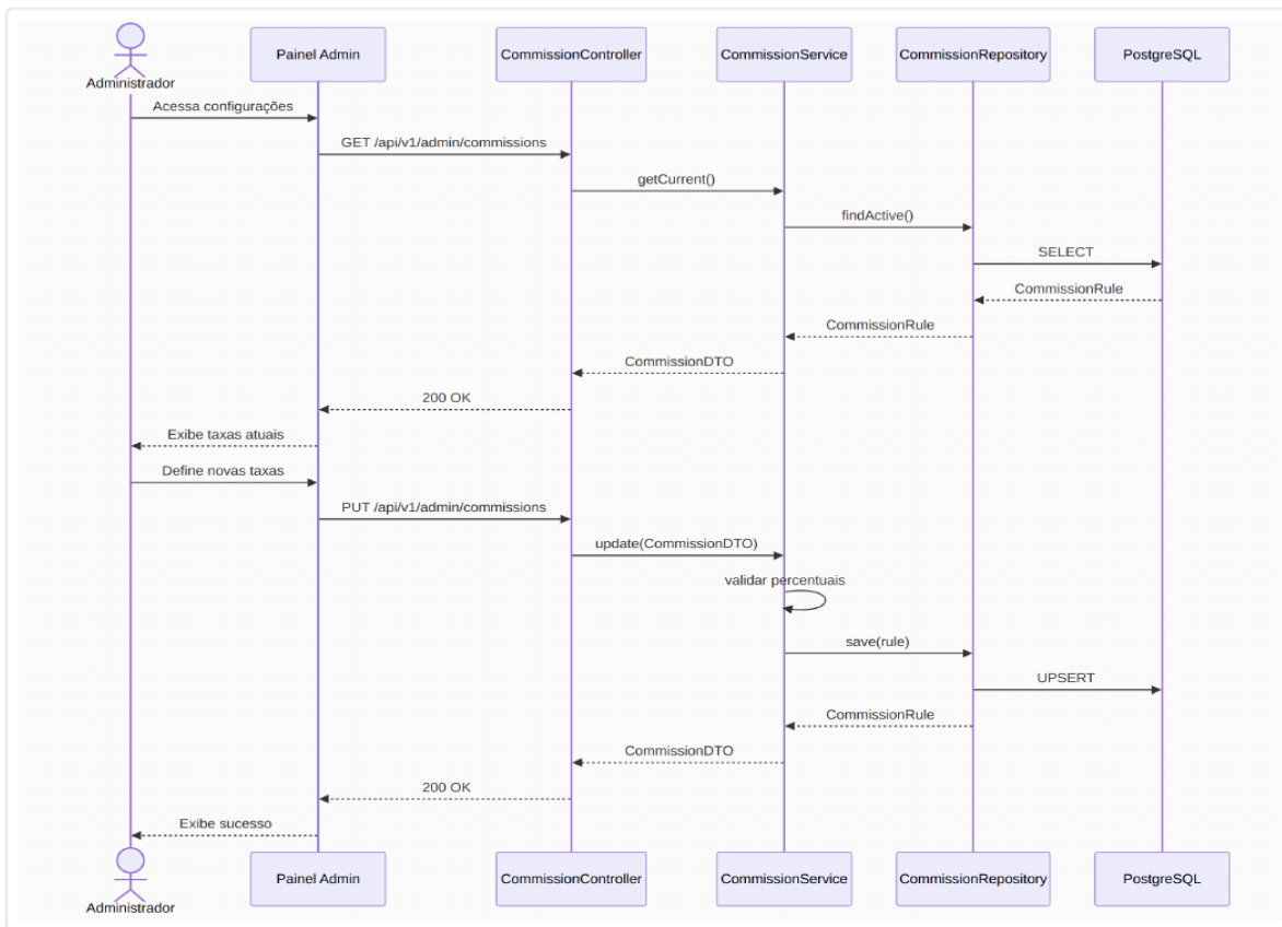
Figura 17 — Diagrama de sequência do UC17 (Configurar taxas de comissão).
