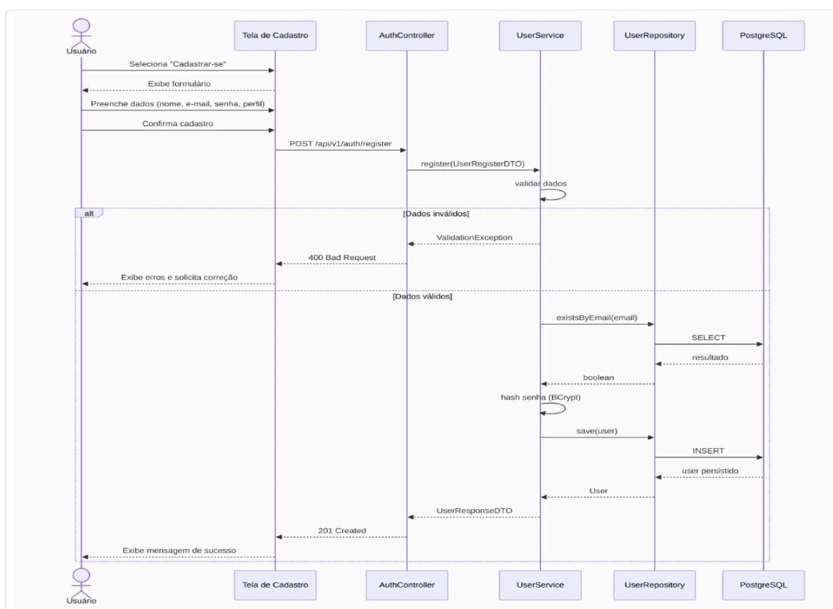
Figura 1 — Diagrama de sequência do UC01 (Cadastrar-se na plataforma).
