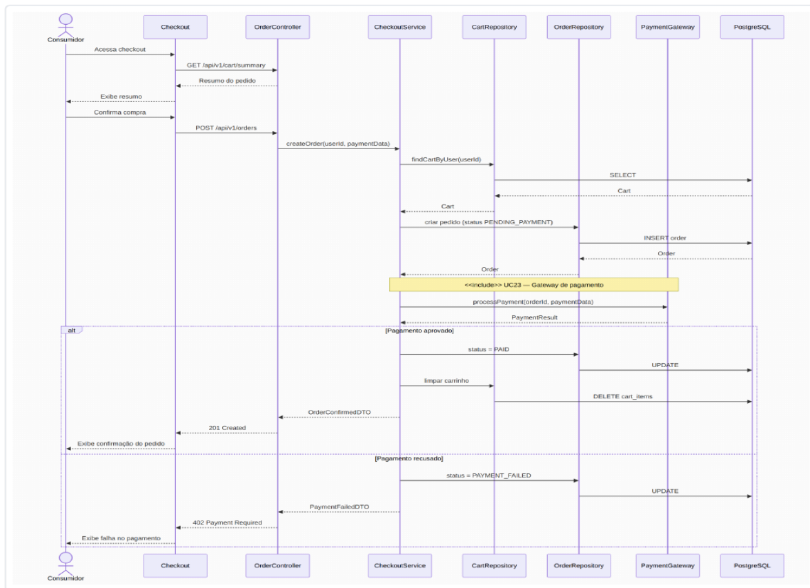
Figura 7 — Diagrama de sequência do UC07 (Realizar checkout).
