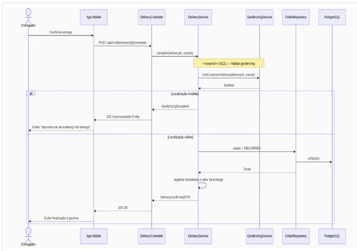
Figura 20 — Diagrama de sequência do UC20 (Confirmar entrega ao consumidor).
