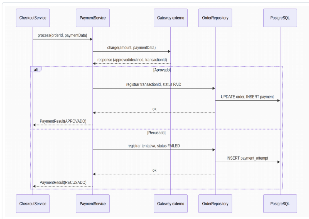
Figura 23 — Diagrama de sequência do UC23 (Gateway de pagamento).
